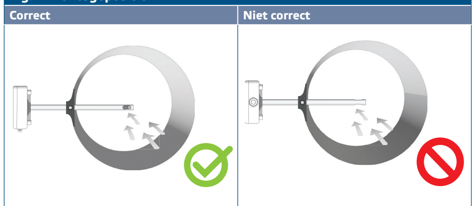
Fig. 2 Montagepositie
