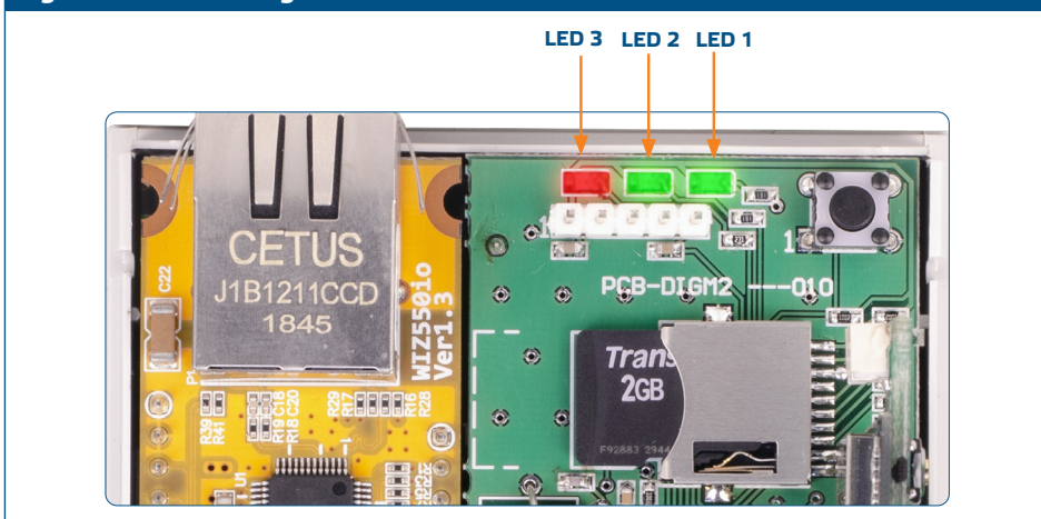
Fig. 6 LED-aanduidingen
