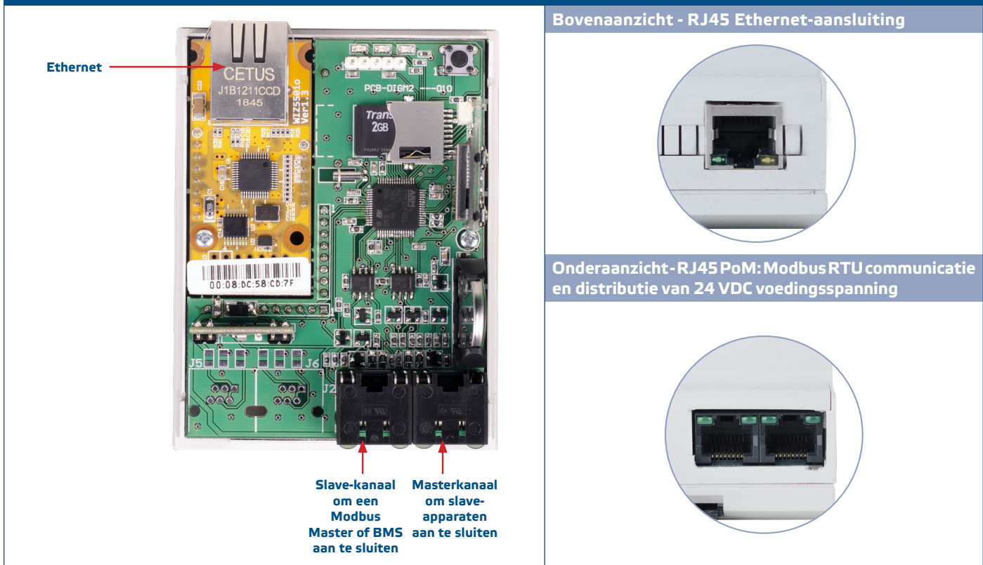
Fig. 3 Aansluitschema
