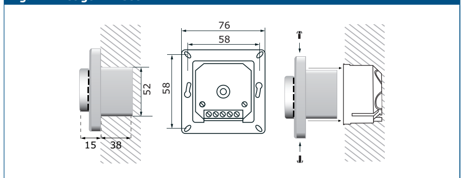
Fig. 2 Afmetingen - inbouw
