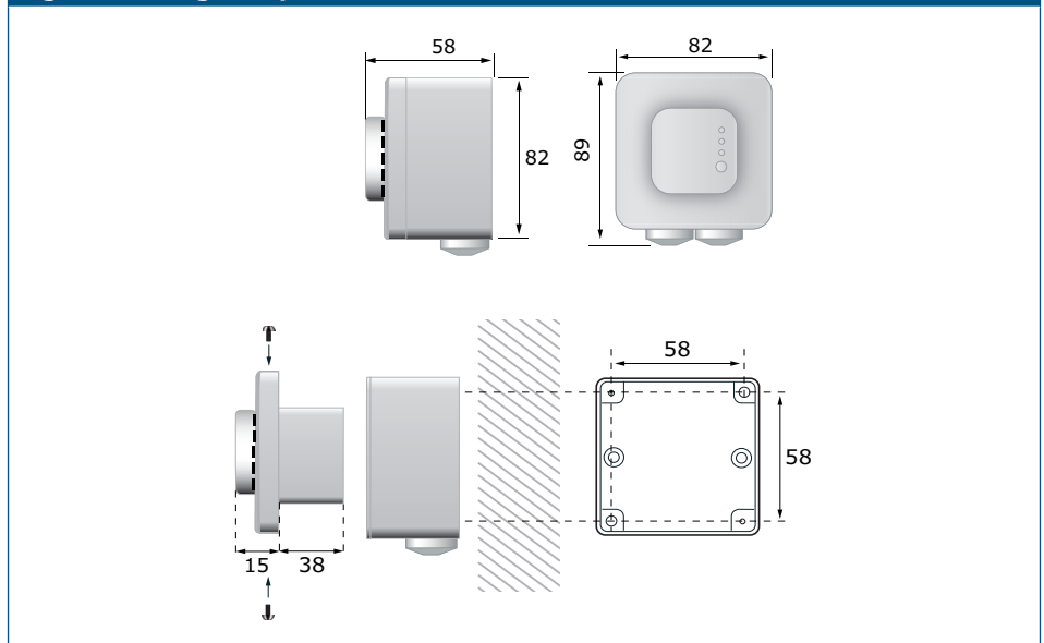
Fig. 3 Afmetingen - opbouw
