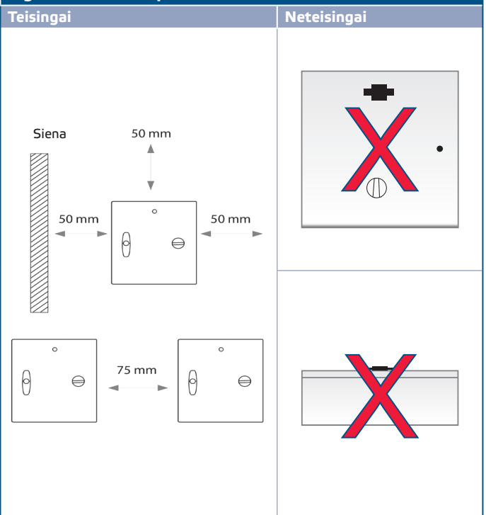
Fig. 2 Montavimo padėtis
