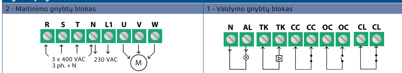
Fig. 3 Pajungimo schema
