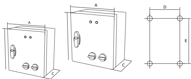
Fig. 1 Montavimo išmatavimai
