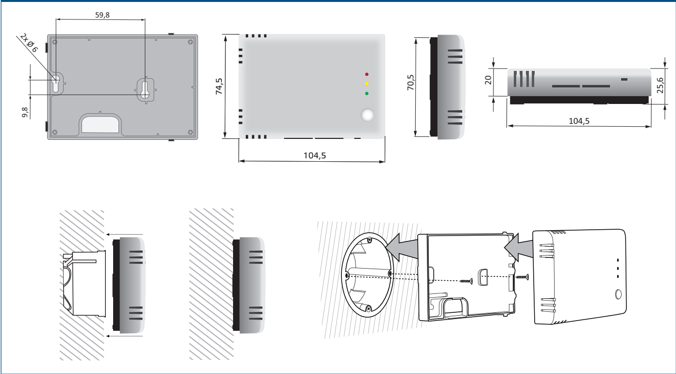
Pav. 2 Montavimo išmatavimai
