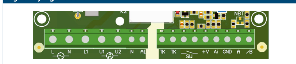
Fig. 3 Pajungimo schema
