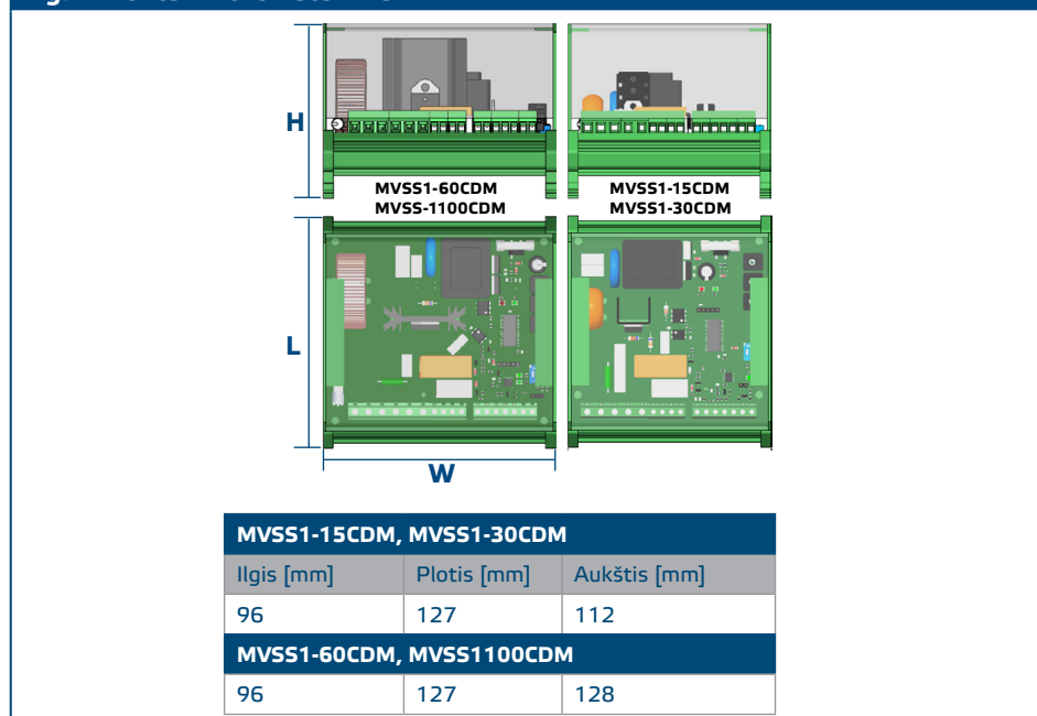
Fig. 1 Montavimo išmatavimai
