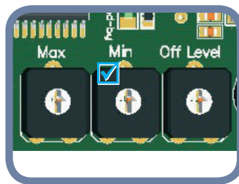
Fig. 7 Min. Greičio trimeris
