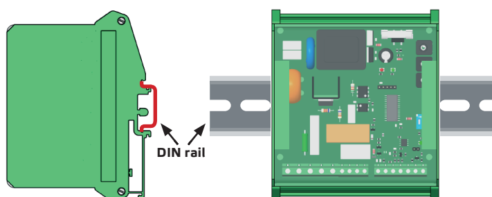
Fig. 2 Montavimo padėtis
