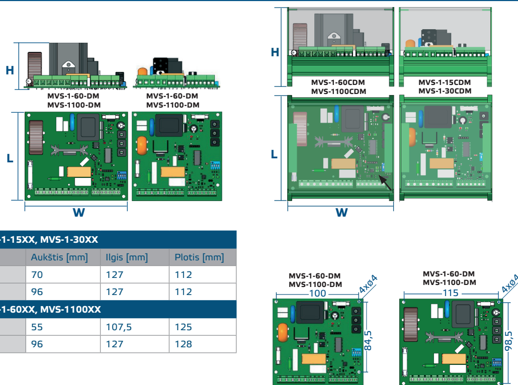
Fig. 1 Montavimo išmatavimai
