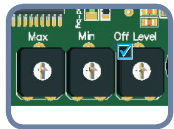
Fig. 8 Išjungimo lygio trimeris
