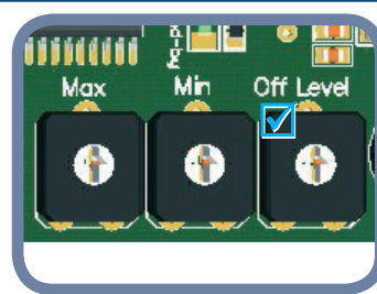
Fig. 8 Išjungimo lygio trimeris
