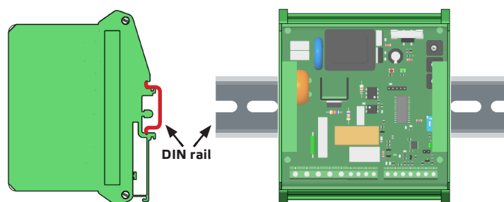
Fig. 2 Montavimo padėtis
