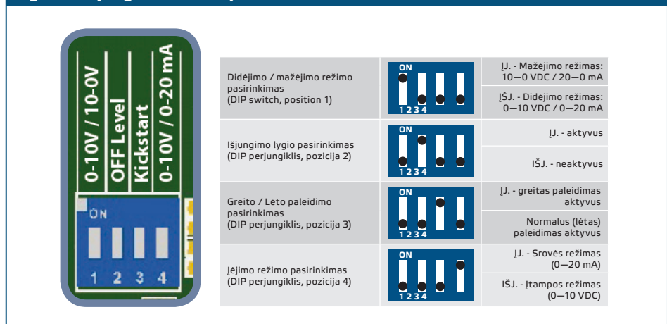
Fig. 4 DIP jungiklio nustatymai
