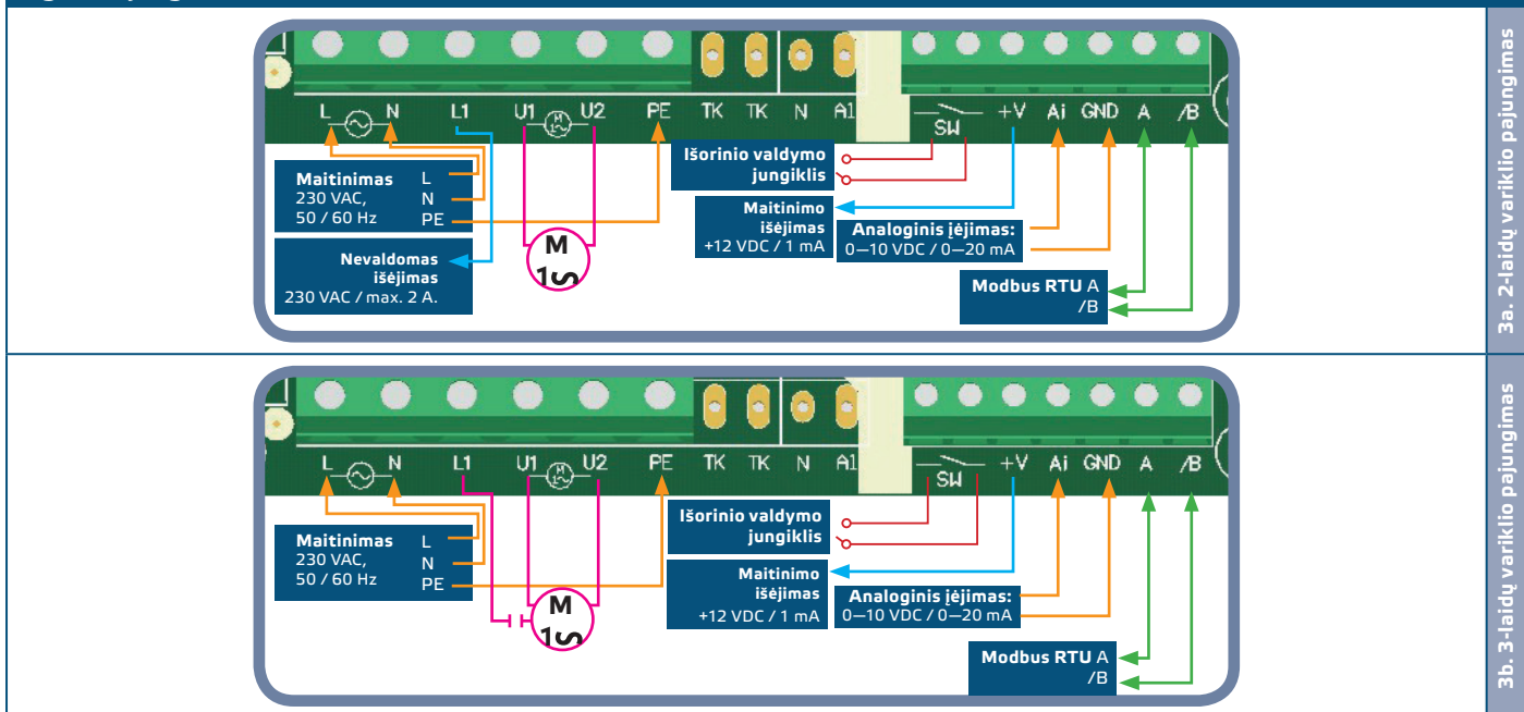
Fig. 3 Pajungimo schema
