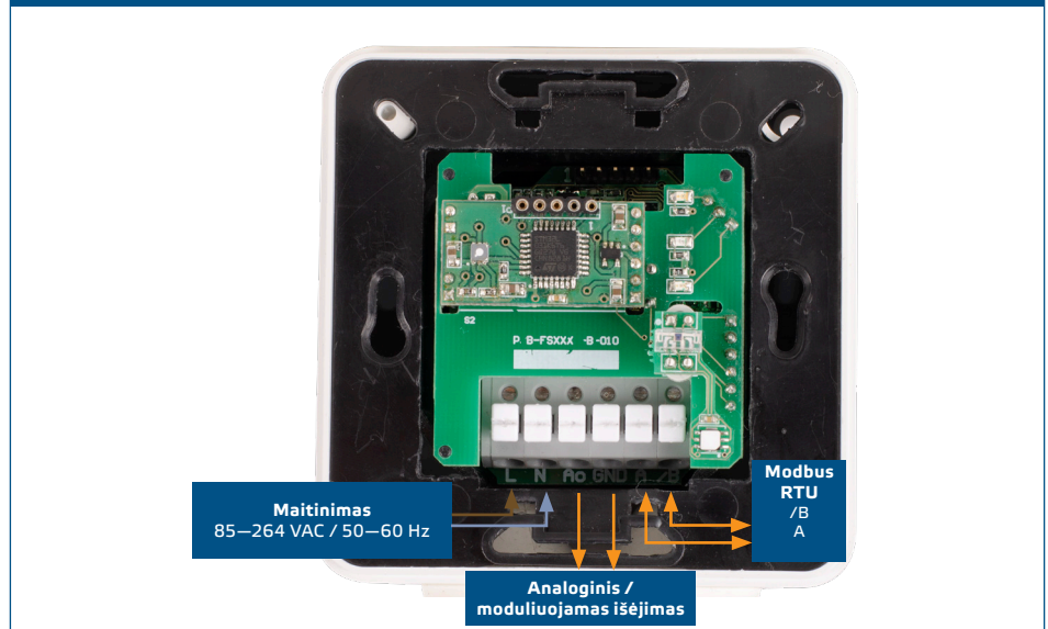
Fig. 1 Pajungimo schema
