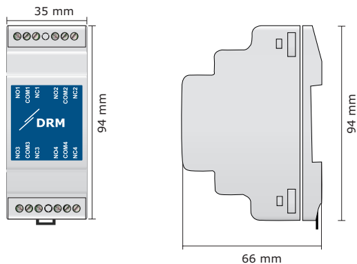
Fig. 1 Montavimo išmatavimai
