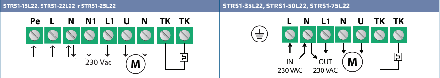
Fig. 3 Pajungimo schema
