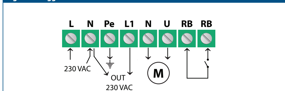
Fig. 3 Cablaggio e connessioni
