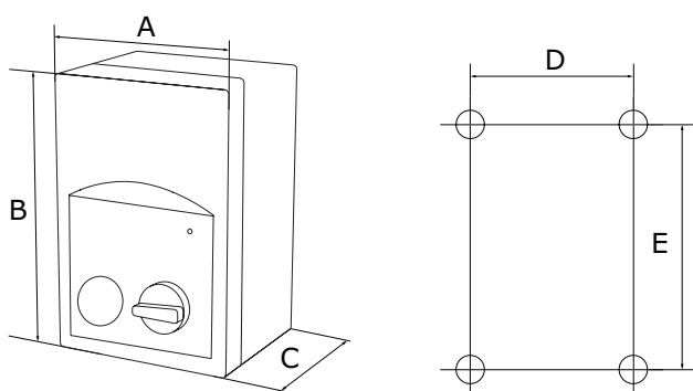
Fig. 1 Dimensioni di montaggio
