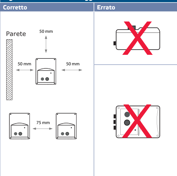
Fig. 2 Posizione di montaggio
