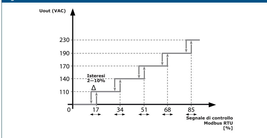
Fig. 4 Modalità automatica "avanti": Velocità da bassa ad alta
