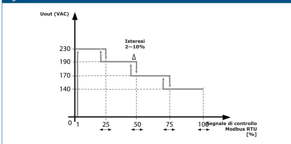
Fig. 5 Modalità automatica "inversione": Velocità da alta a bassa
