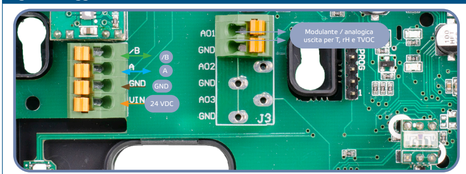
Fig. 4 Cablaggio
