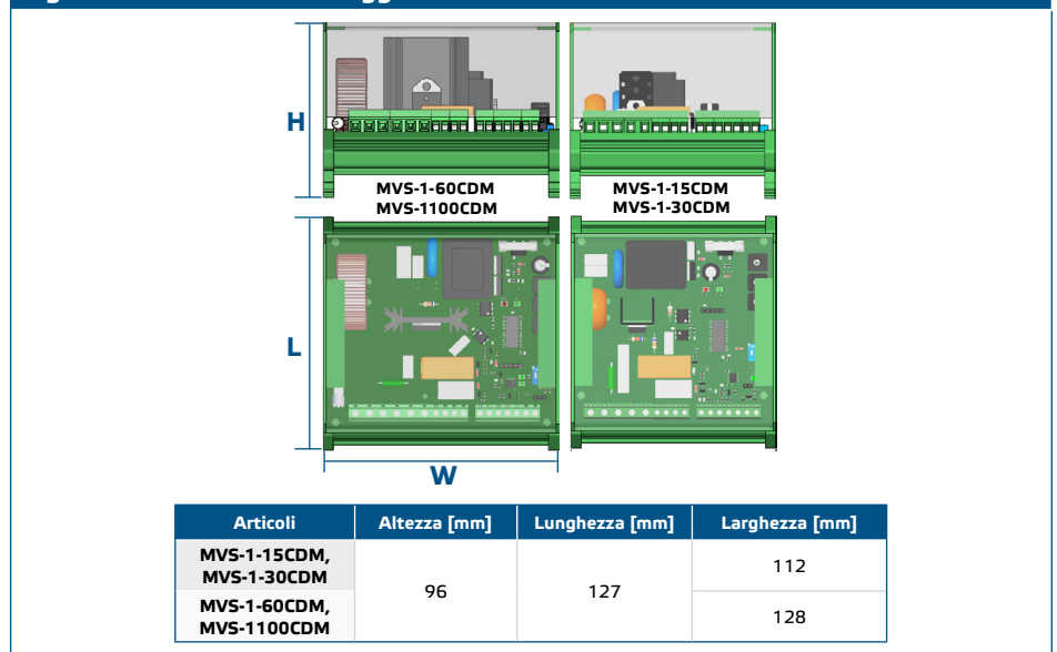
Fig. 1 Dimensioni di montaggio
