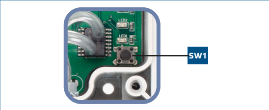
Fig.6 Calibrazione del sensore e reset del registro Modbus
