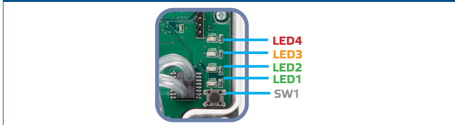
Fig. 9 Indicazioni LED
