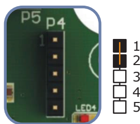
Fig. 8 Ponticello di ripristino del registro di mantenimento Modbus
