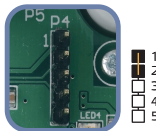
Fig. 8 Ponticello di ripristino del registro di mantenimento Modbus
