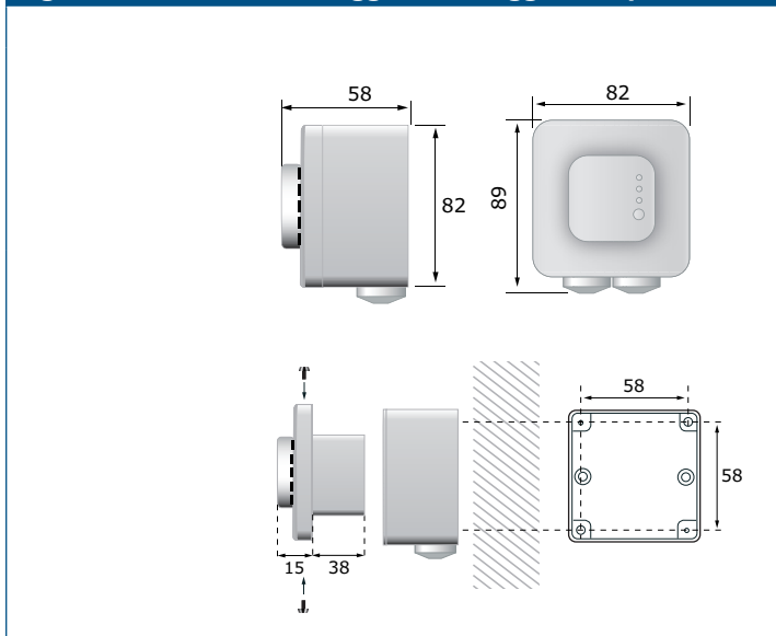
Fig. 4 Dimensioni di montaggio - montaggio in superficie
