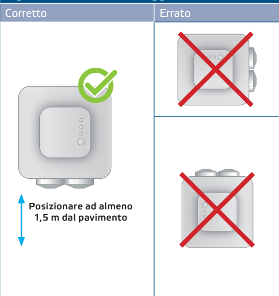
Fig. 5 Posizione di montaggio
