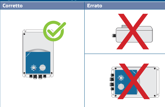
Fig. 2 Posizione di montaggio
