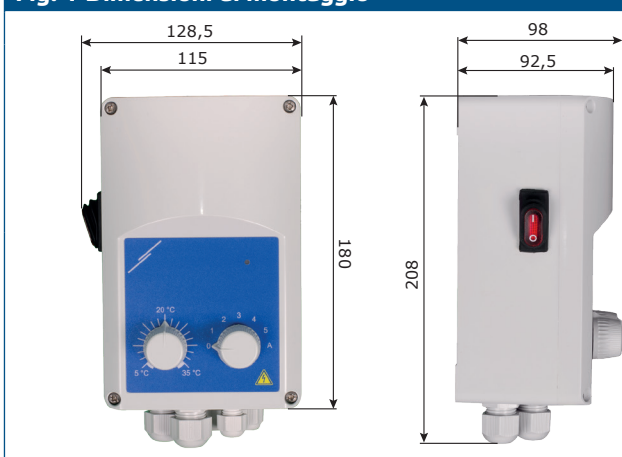
Fig. 1 Dimensioni di montaggio
