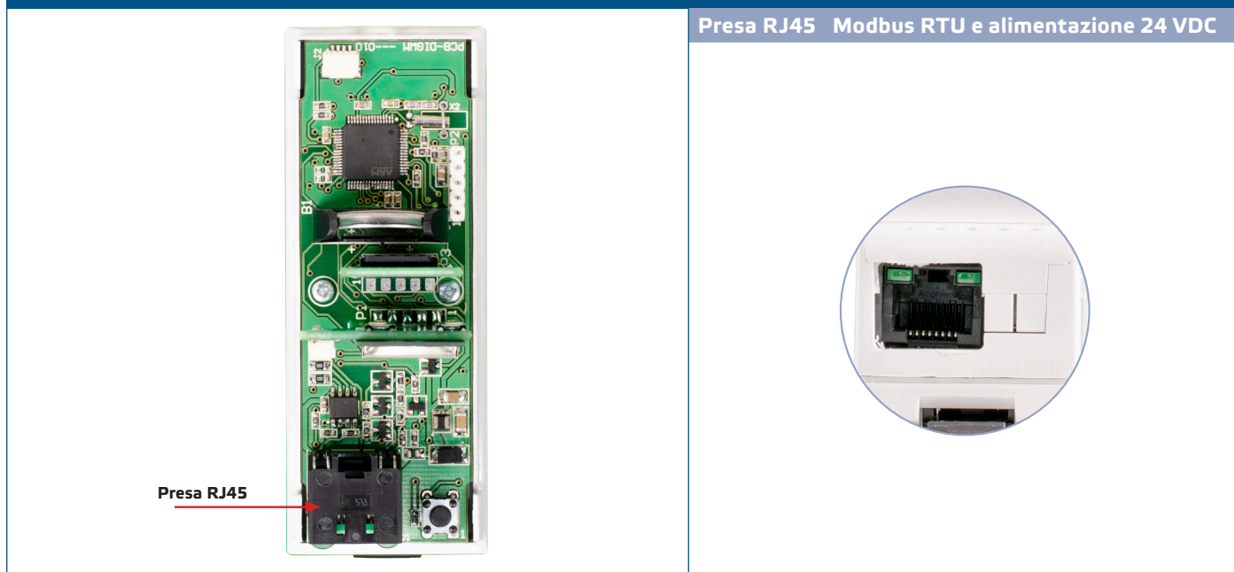
Fig. 3 Cablaggio e connessioni
