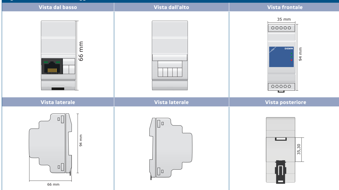
Fig. 2 Posizione di montaggio
