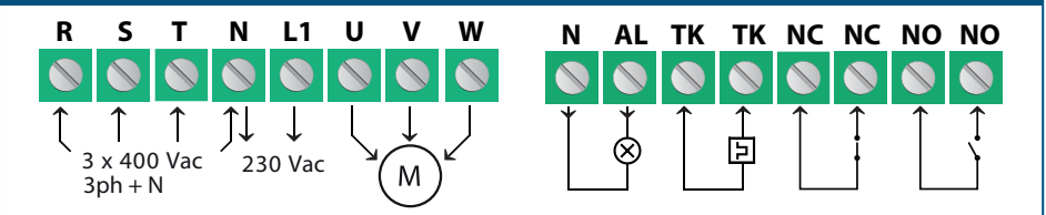
Fig. 3 Cablaggio e connessioni
