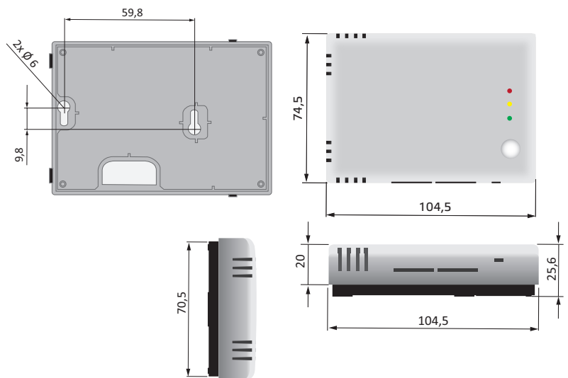
Fig. 2 Dimensions de montage
