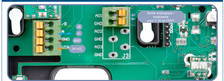
Fig. 4 Câblage
