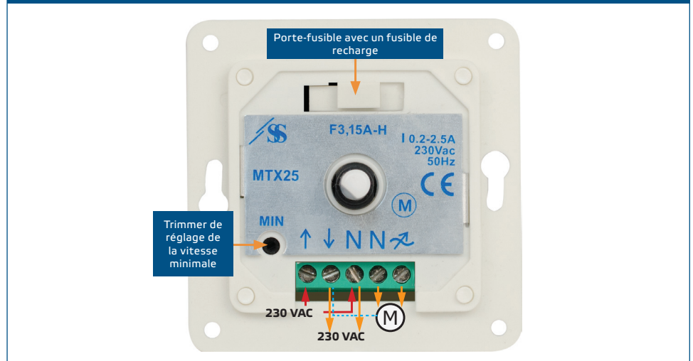
Fig. 1 Câblage et raccordements
