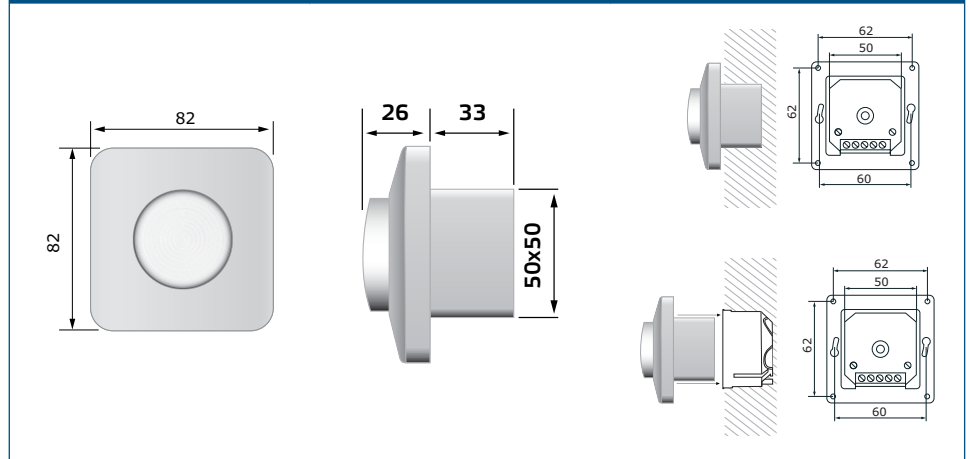
Fig. 2 Dimensions de montage – montage encastré
