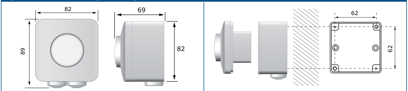
Fig. 3 Dimensions de montage – montage en saillie
