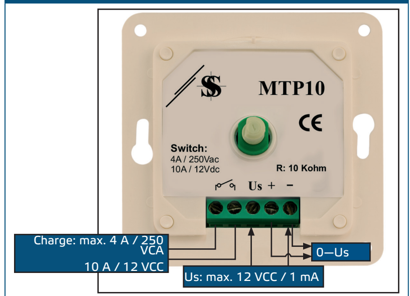
Fig. 1 Câblage et raccordements
