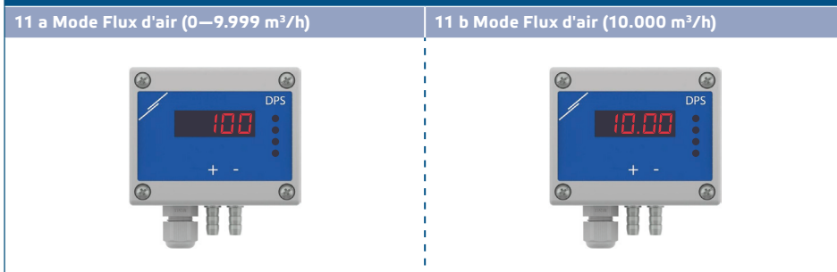
Fig. 11 Affichage du mode Flux d'air et du mode Vitesse d'air
