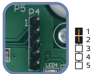
Fig. 8 Cavalier de réinitialisation des registres Modbus
