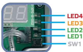
Fig. 6 Etalonnage du capteur et réinitialisation des registres Modbus
