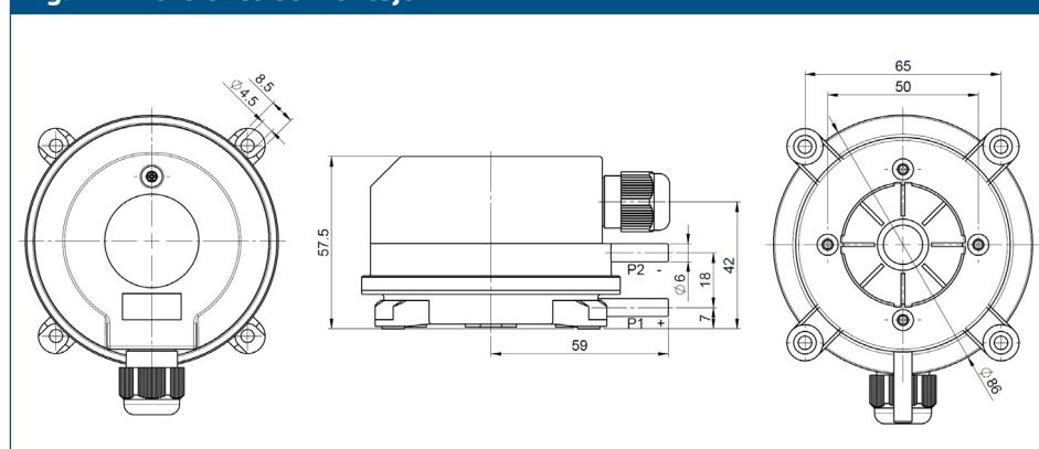
Fig. 2 Dimensiones de montaje
