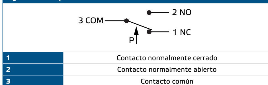
Fig. 1 Cableado y conexiones
