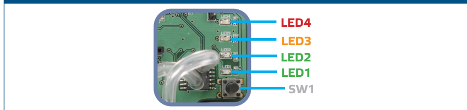
Fig. 10 Indicaciones LED de calibración y de reinicio del registro Modbus
