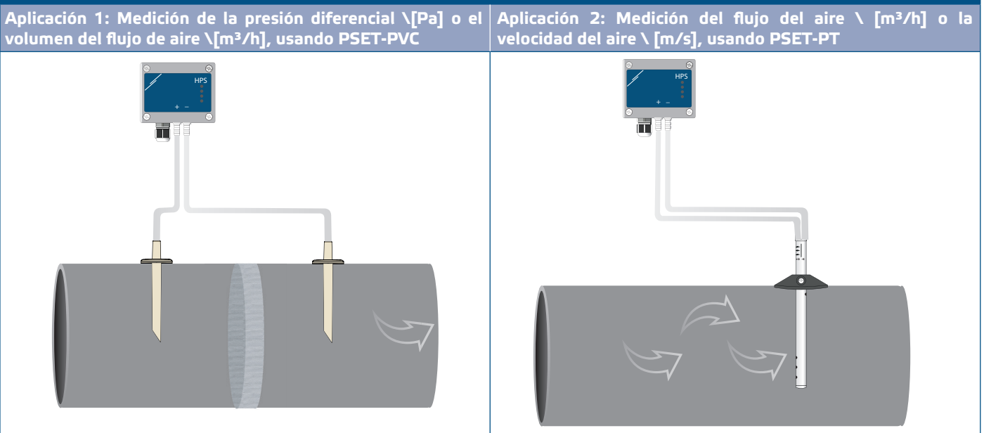
Fig. 4 Conexión al conducto
