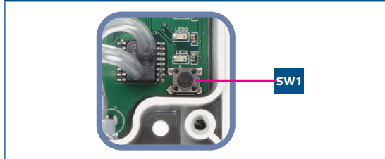
Fig. 8 Calibración del sensor y reinicio del registro Modbus
