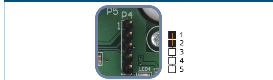
Fig. 11 'Jumper' de reinicio de los 'holding registers'
