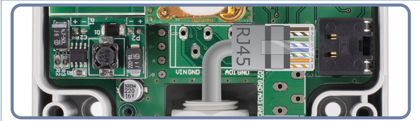
Fig. 4 Cableado y conexiones
