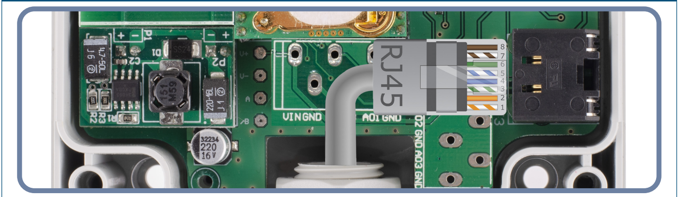
Fig. 4 Cableado y conexiones
