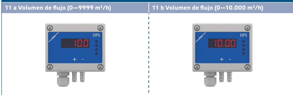
Fig. 11 Modo de visualización de los valores medidos de volumen de flujo
