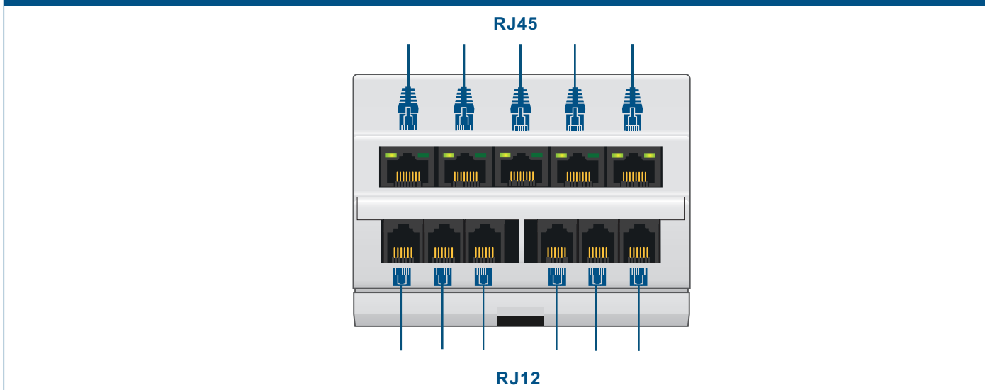
Fig. 4 Conexiones RJ45 y RJ12
