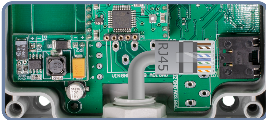
Fig. 4 Cableado y conexiones
