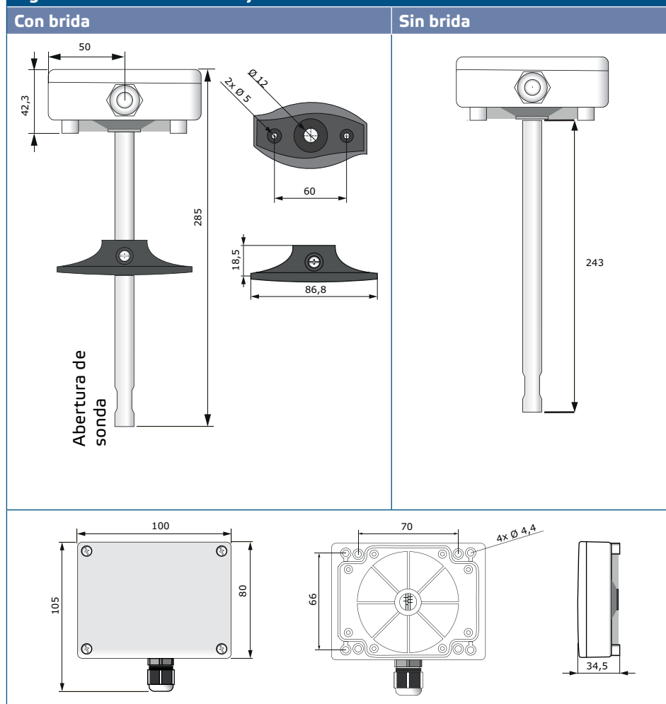
Fig. 1 Dimensiones de montaje
