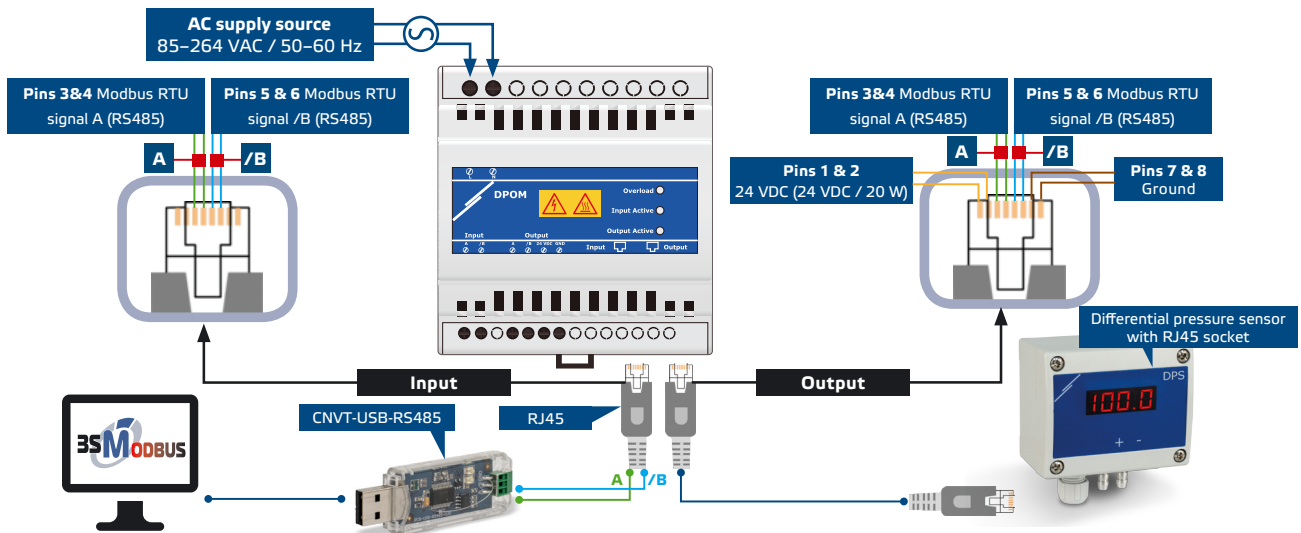
Fig. 3 Wiring diagram
