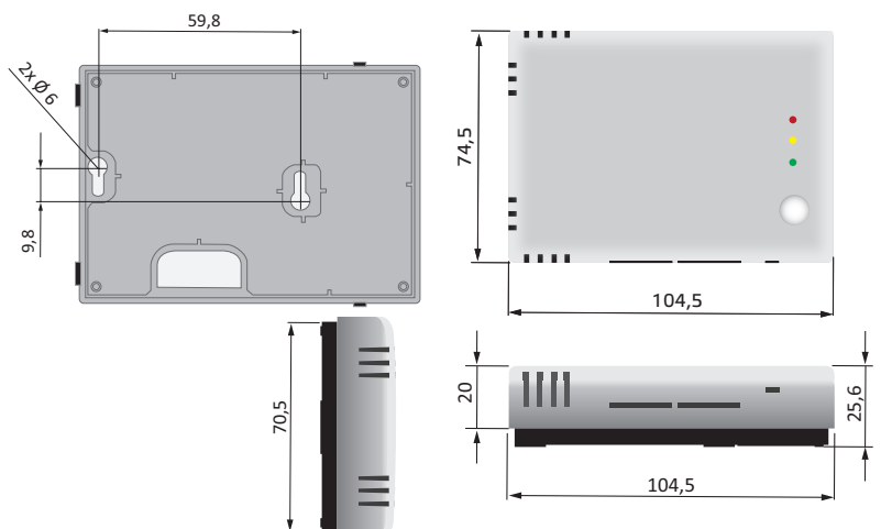
Fig. 2 Einbaumaße
