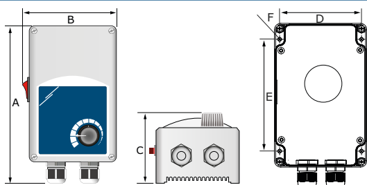
Fig. 1 Einbaumaße
