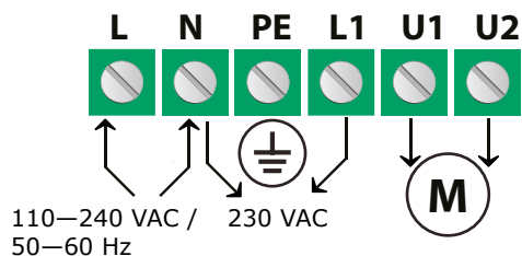
Fig. 3 Verdrahtung und Anschlüsse
