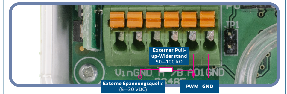
Fig. 6 PWM ( offener Kollektor ) Anschluss (JP1 nicht verbunden)
