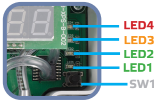
Fig. 8 Sensorkalibrierungsverfahren und Modbus-Register Reset Taktschalter und Anzeigen
