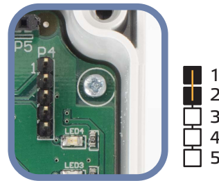
Fig. 10 Modbus Holding Register Reset Steckbrücke
