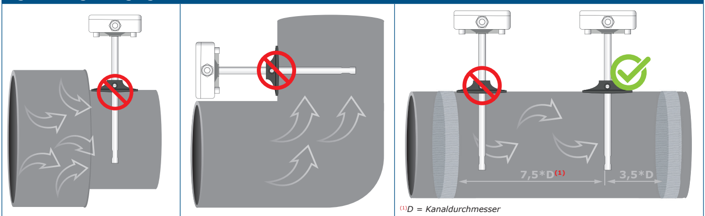
Fig. 3 Montagebedingungen
