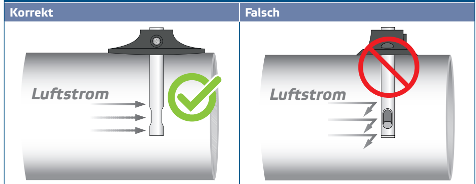
Fig. 2 Einbaulage
