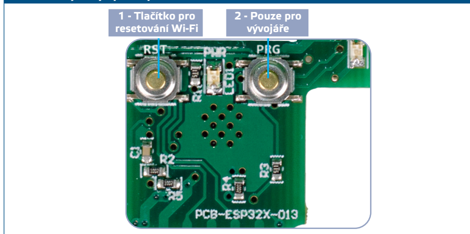
Obr. 5 Dotykový spínač pro resetování Wi-Fi
