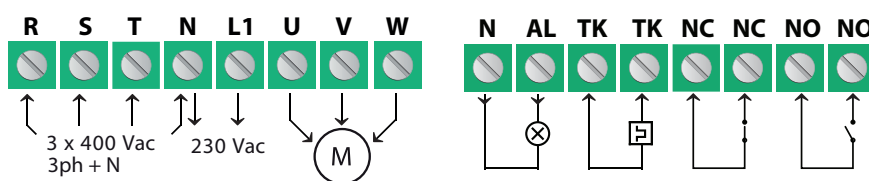
Obr. 3 Elektroinstalace a připojení
