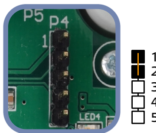
Obr. 8 Propojka pro resetování holding registru Modbus
