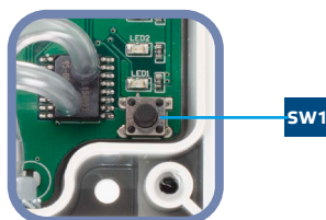
Obr. 6 Kalibrace čidla a reset registru Modbus
