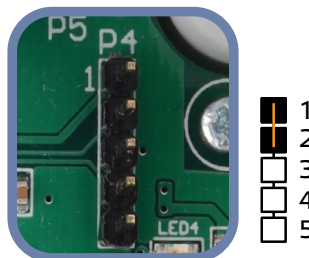
Obr. 8 Propojka pro resetování holding registru Modbus
