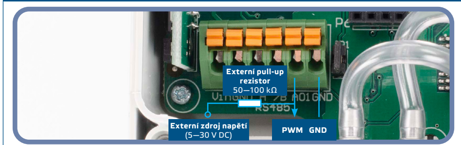
Obr. 6 Připojení PWM (Open collector)
