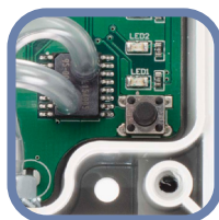
Obr. 8 Indikace kalibrace čidla a resetovací spínač registru Modbus
