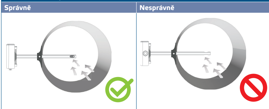
Obr. 2 Montážní poloha
