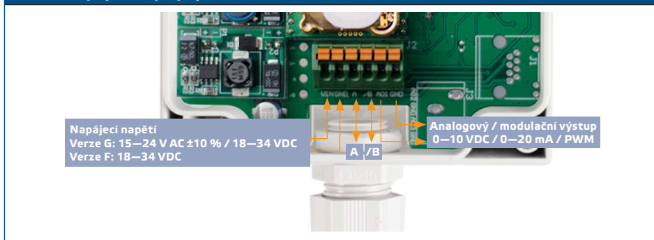
Obr. 4 Zapojení a připojení
