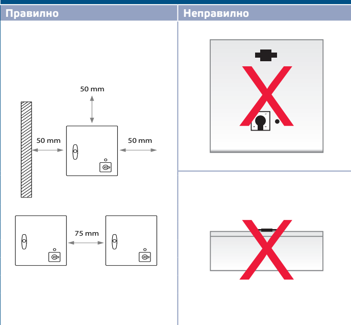
Фиг. 2 Положение за монтаж
