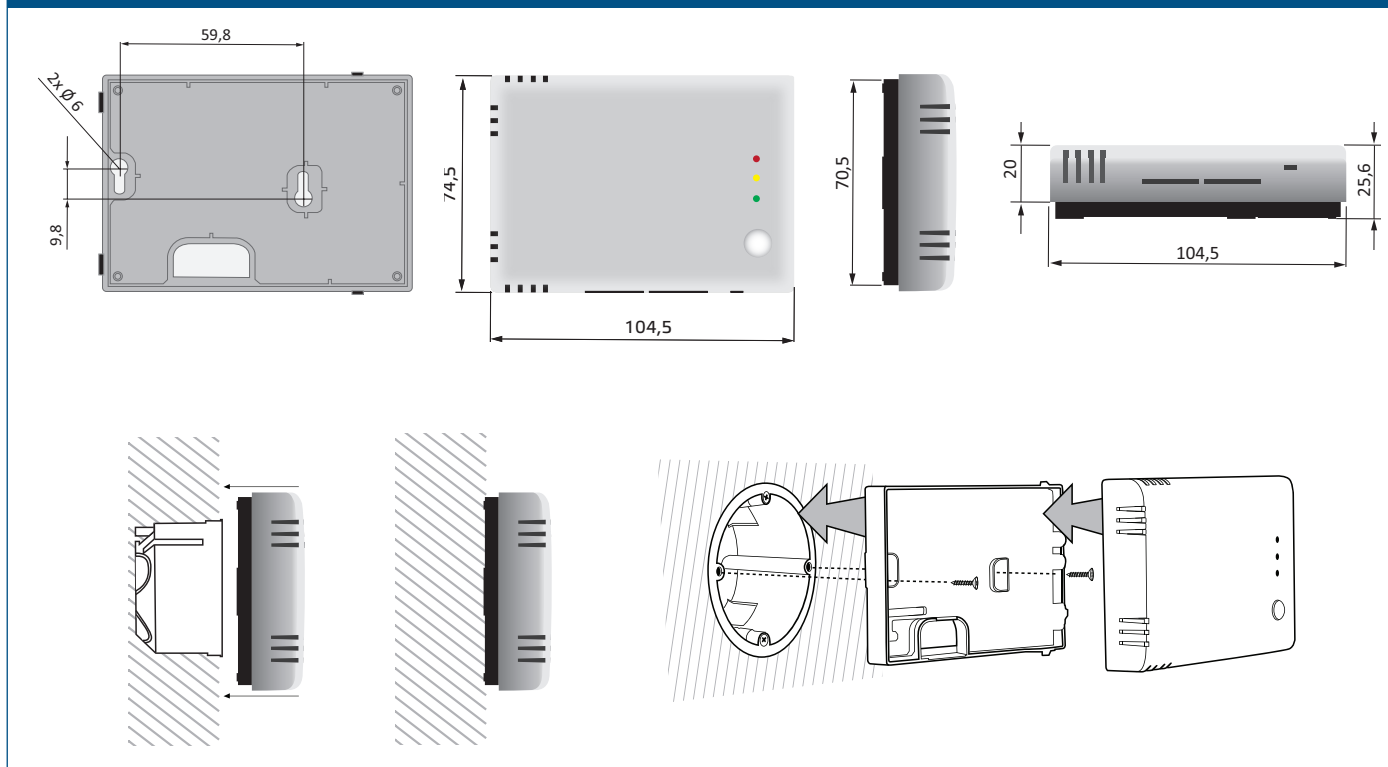
Фиг. 2 Монтажни размери
