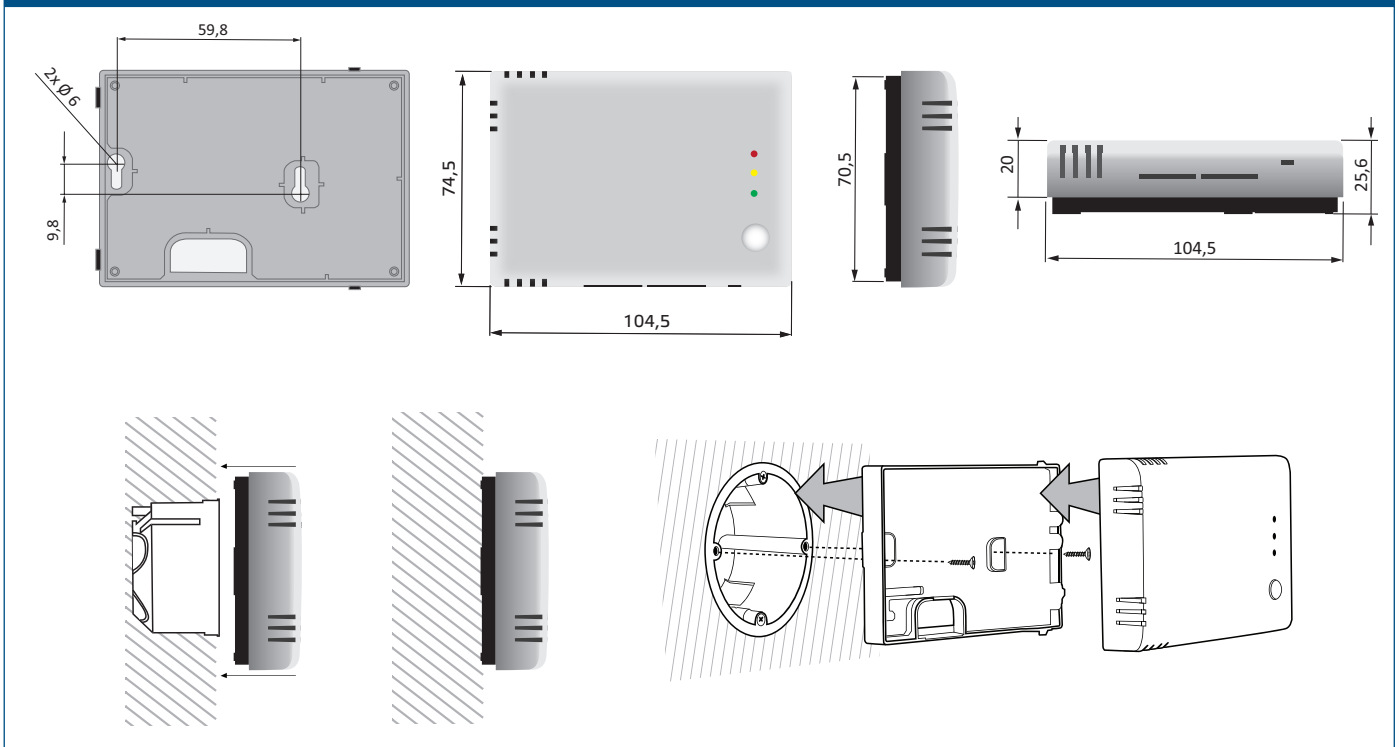
Фиг. 2 Монтажни размери
