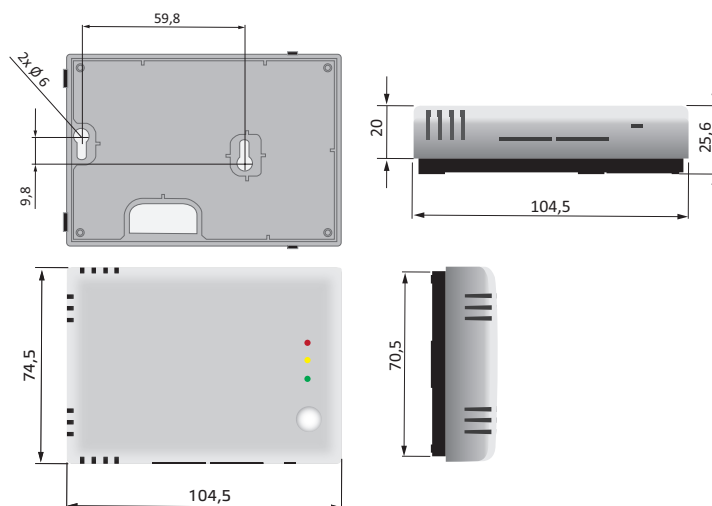
Фиг. 2 Монтажни размери
