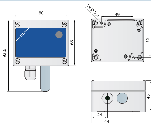
Fig. 1 Монтажни размери
