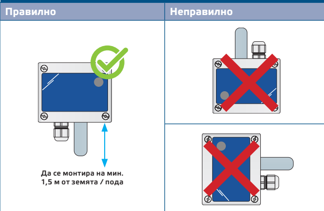
Fig. 2 Монтажна позиция
