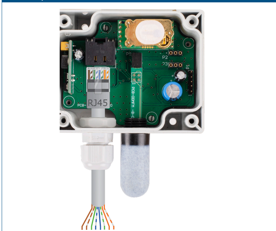
Фиг. 3 Свързване
